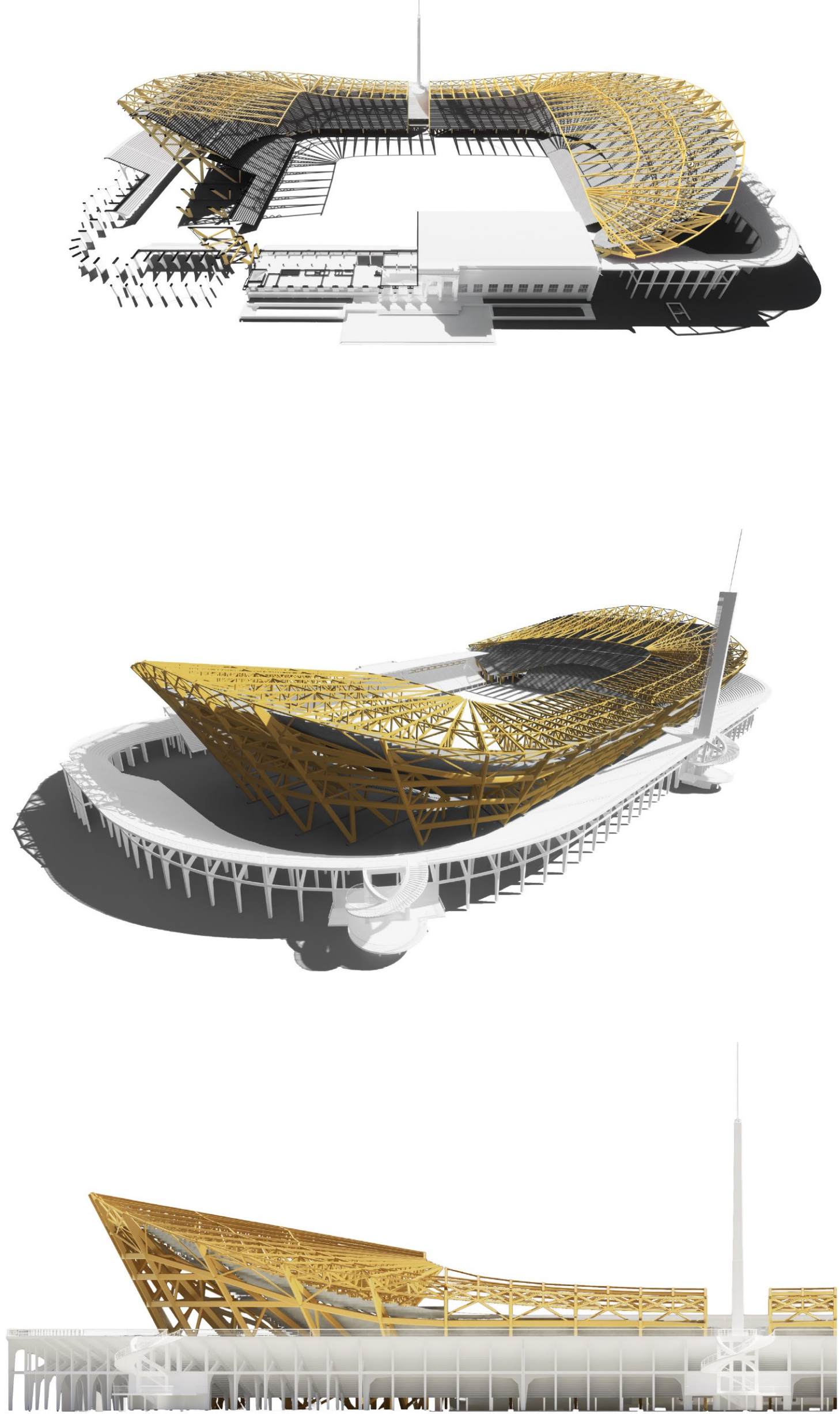
Rendering Strutturali | Simulazioni BIM
