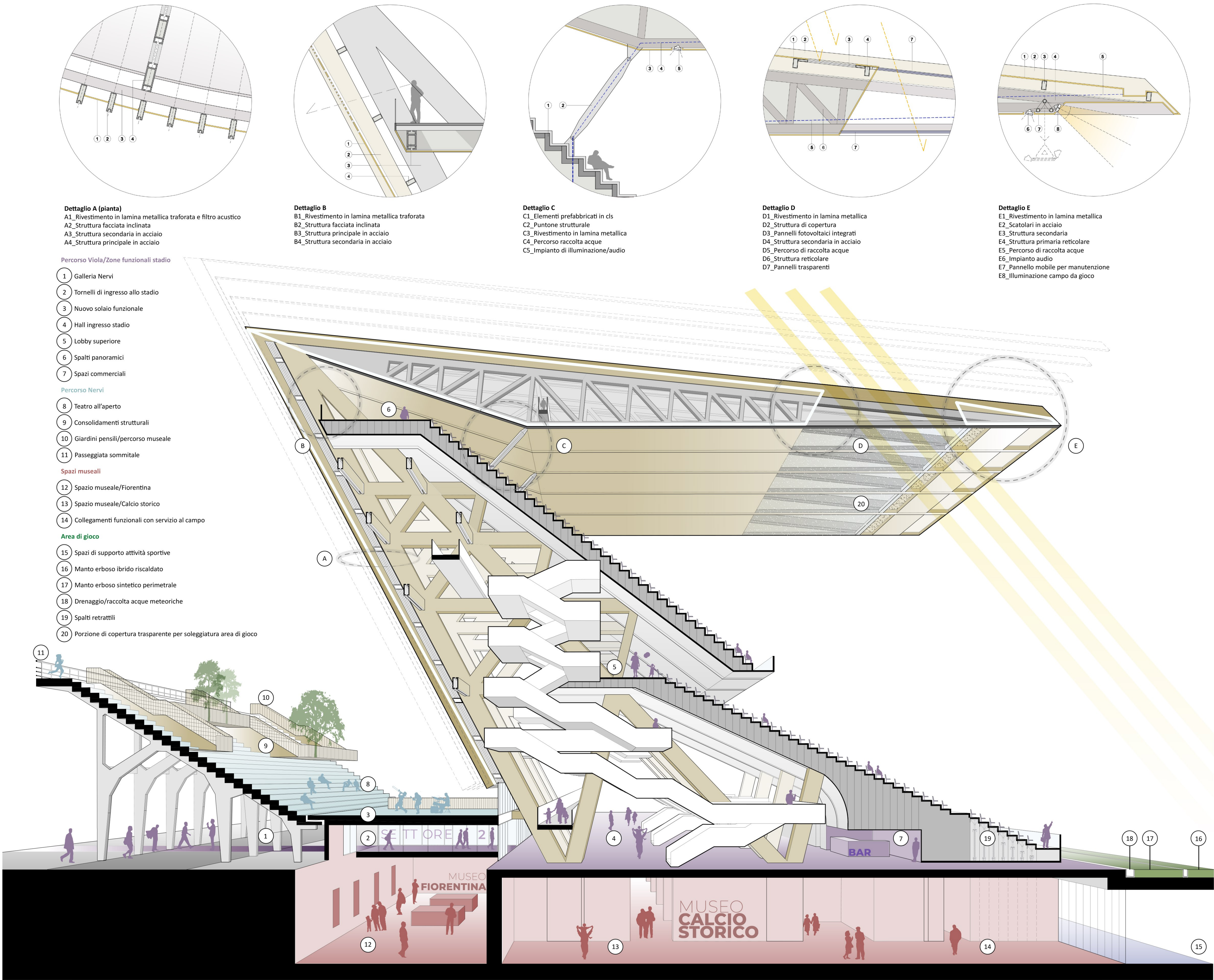
Sezione Prospettica | Rispetto e valorizzazione dell'immagine complessiva dell'opera di Pier Luigi Nervi e coerenza architettonica di nuove aggiunte
